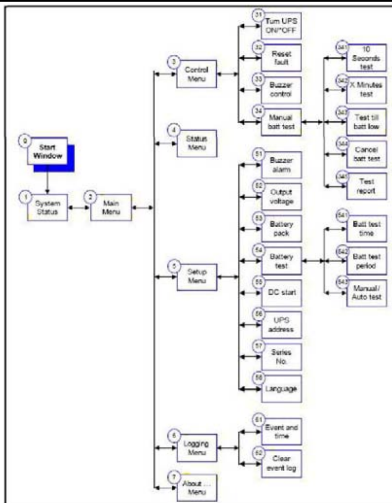
Рисунок 4-3. Структура меню
