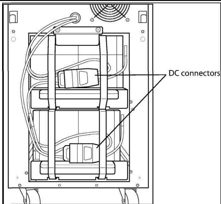
Рисунок 5-2. Отсоединение лотка и аккумуляторных батарей
