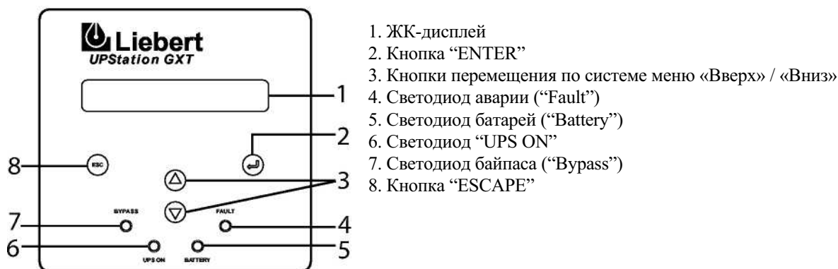
Рисунок 4-2. Панель управления
