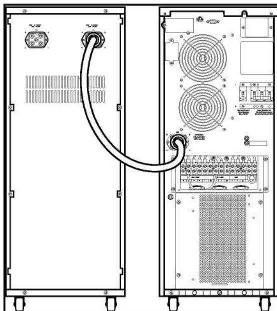
Рисунок 3-6. ИБП GXT2 10000T230 с внешним блоком батарей
