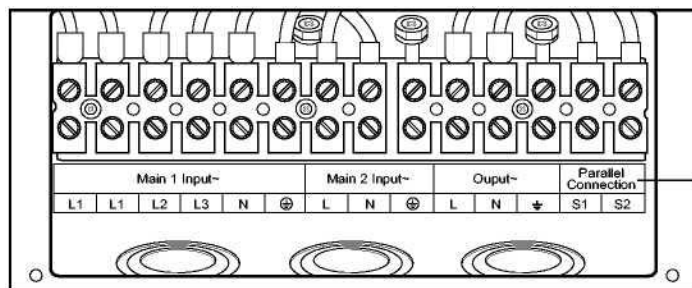
Рисунок 3-5. Соединители для подключения проводов
