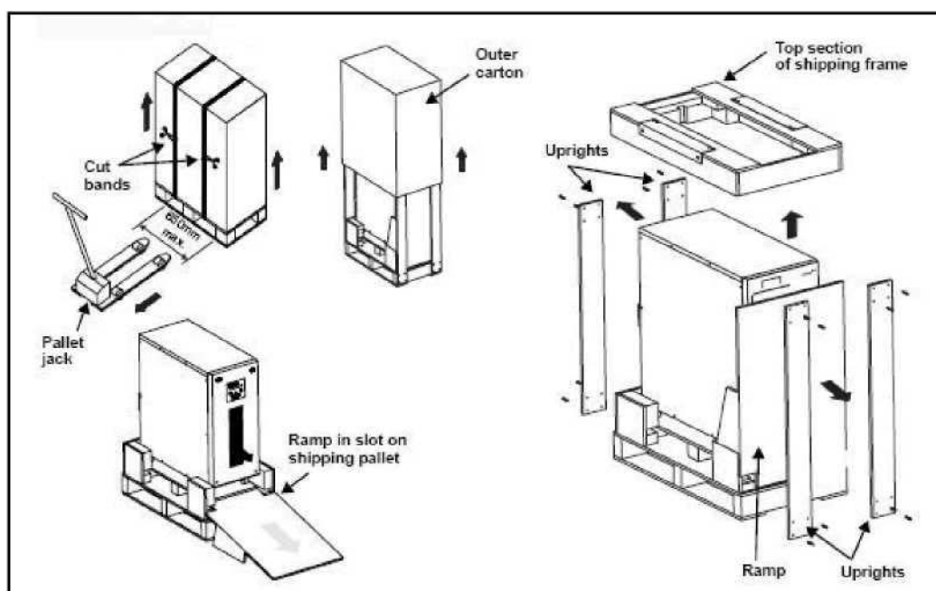
Рисунок 2-1. Распаковка
