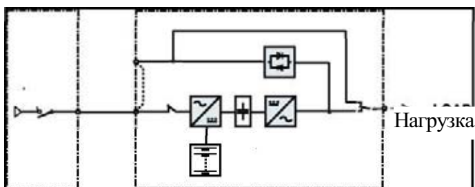
Рисунок 3-3. Стандартная конфигурация – подключение УЗО
