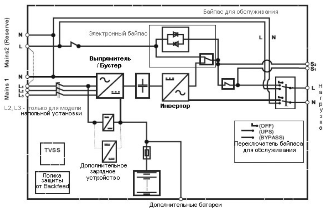
Рисунок 4-1. Блок-схема ИБП модели напольной установки
